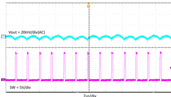
图 7-11. TPS563206 输出电压纹波 (3A 负载)
