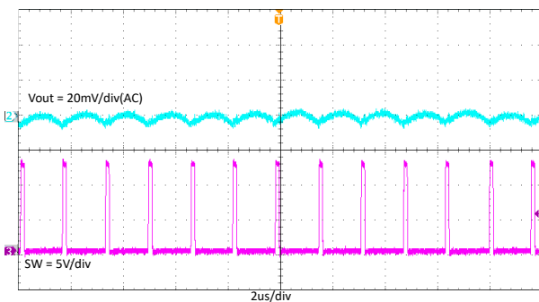
图 7-9. TPS563206 输出电压纹波 (0.1A 负载)
