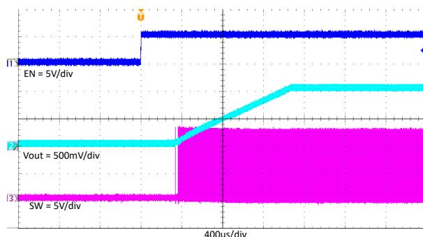
图 7-14. TPS563206 在负载电流为 3A 时使能开
