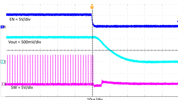
图 7-15. TPS563206 在负载电流为 3A 时使能关
