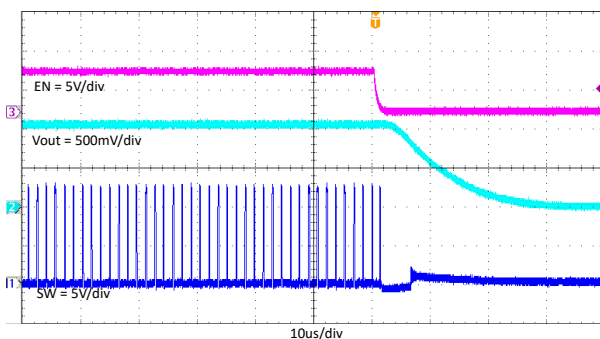
图 7-13. TPS563203 在负载电流为 3A 时使能关
