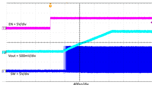
图 7-12. TPS563203 在负载电流为 3A 时使能开
