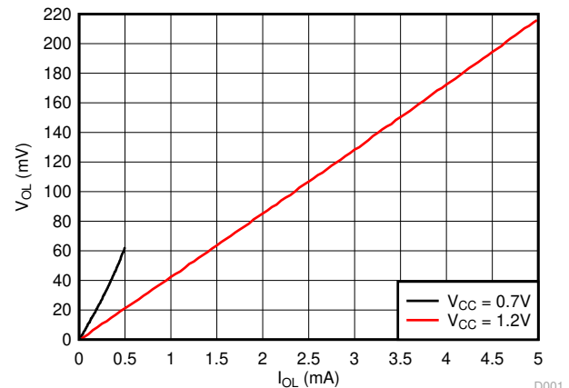
图 5-4. 典型 ( T_A=25^\circ\text{C} ) 输出低电压 ( V_{OL} ) 与灌电流 ( I_{OL} ) 间的关系
