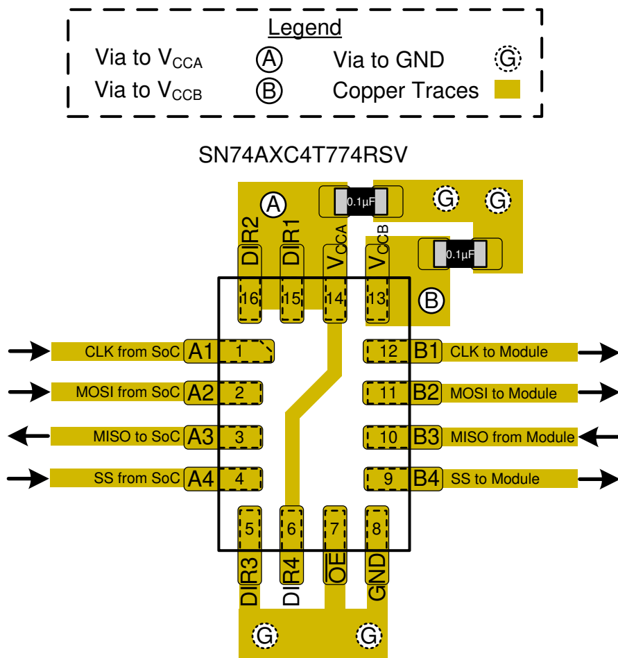
图 8-3. 布局示例
