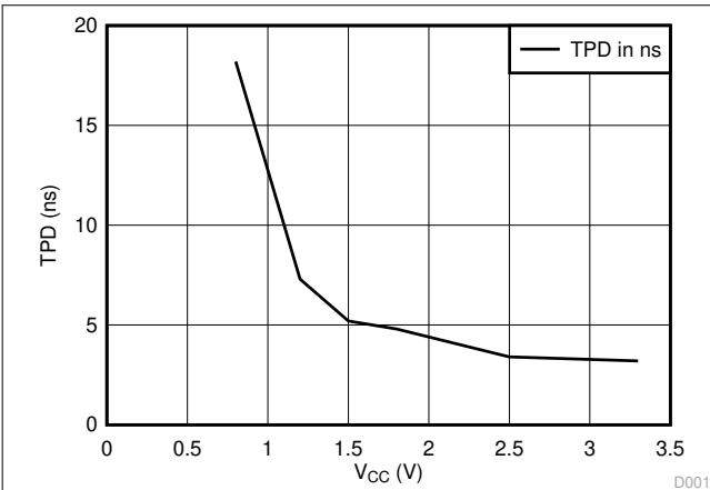
图 6-1. TPD vs V_{CC}
