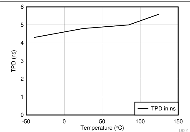
图 6-2. TPD vs Temperature
