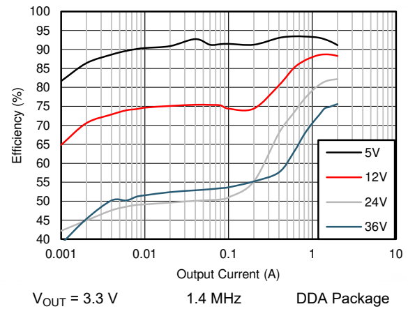
图 9-10. Efficiency
