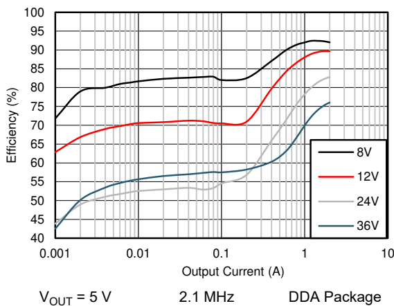
图 9-11. Efficiency
