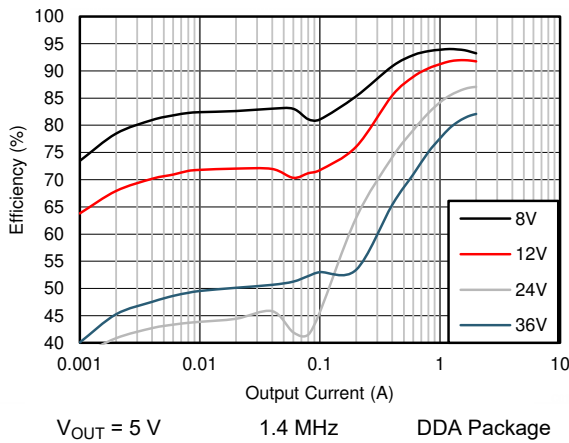
图 9-9. Efficiency
