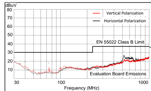
辐射发射图
