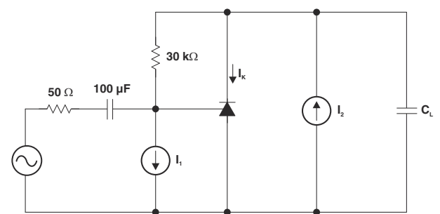
图 5-14. Phase Margin Test Circuit
