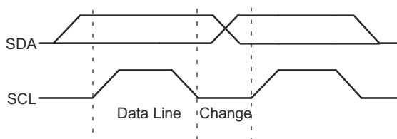
图 7-5. Bit Transfer
