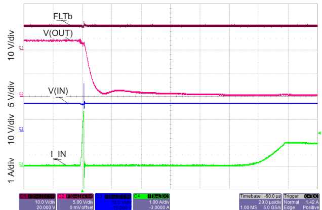
12V 短路响应
