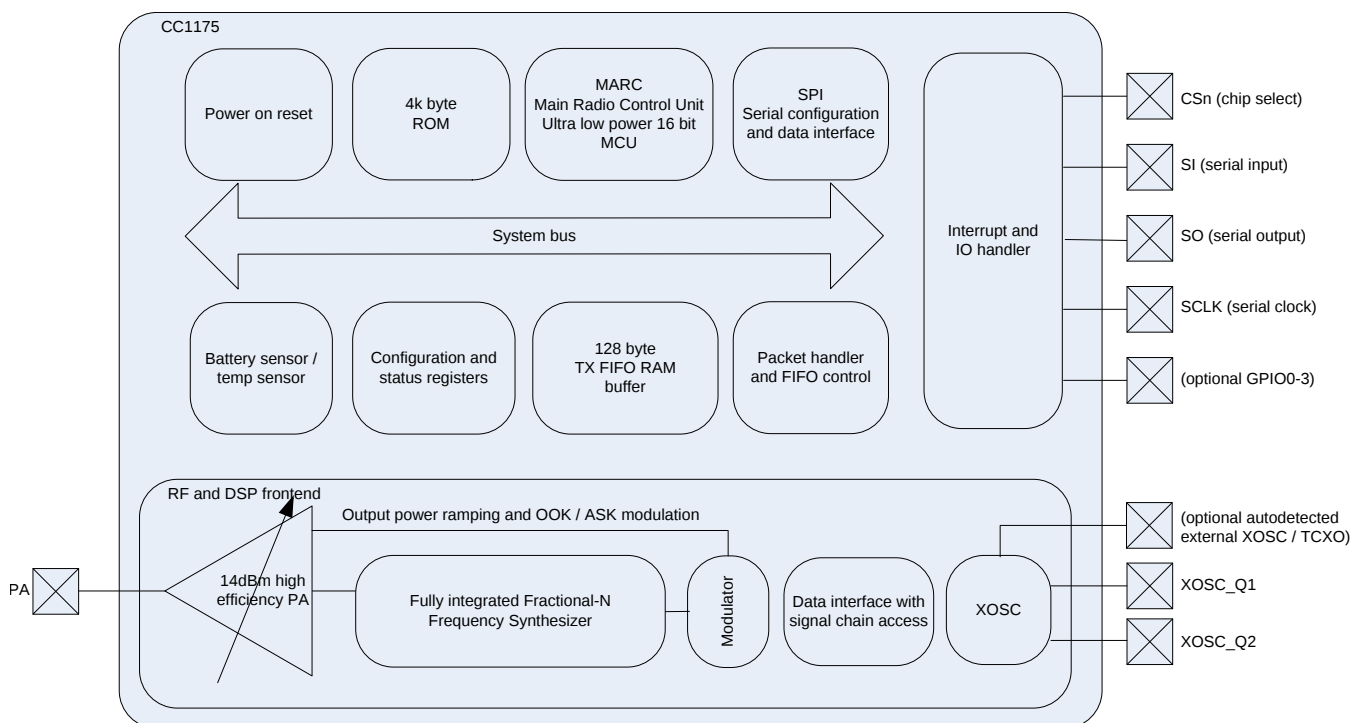
图 1-1. 功能方框图
