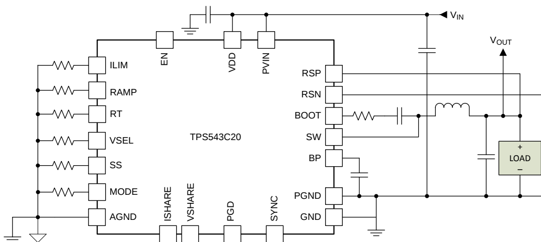
简化原理图
