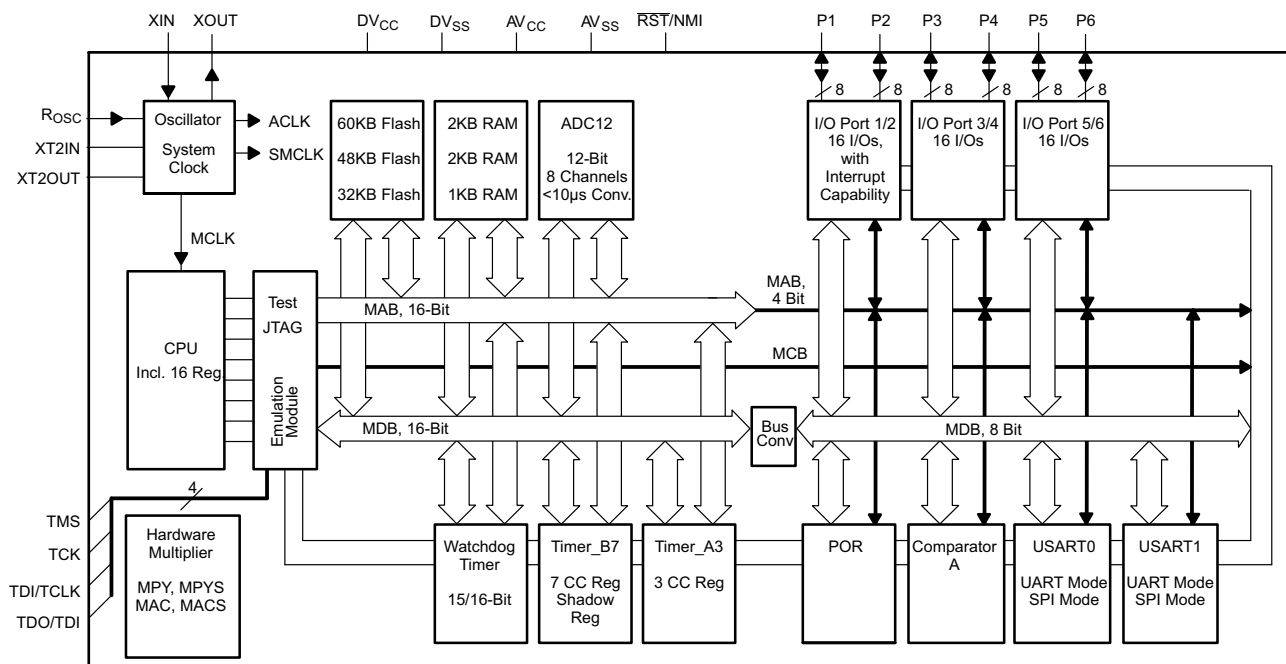
图 1-2. 功能方框图, MSP430F14x
