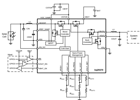
典型应用原理图
