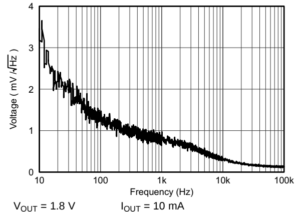
图 25. Output Spectral Noise Density
