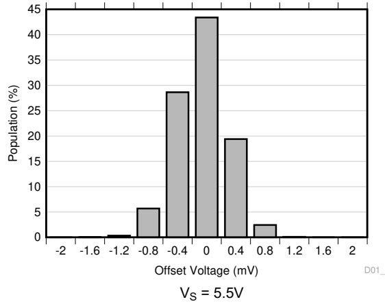
图 7-1. 失调电压分布直方图
