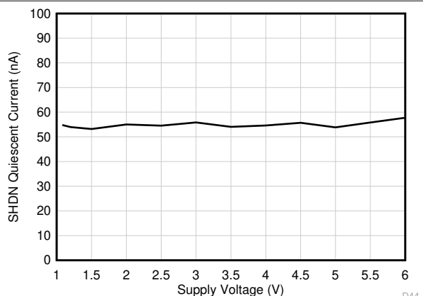
图 7-41. 关断模式静态电流与电源电压间的关系
