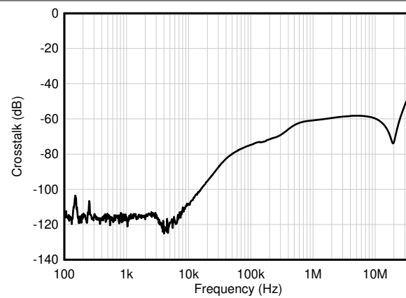
图 7-46. 通道分离
