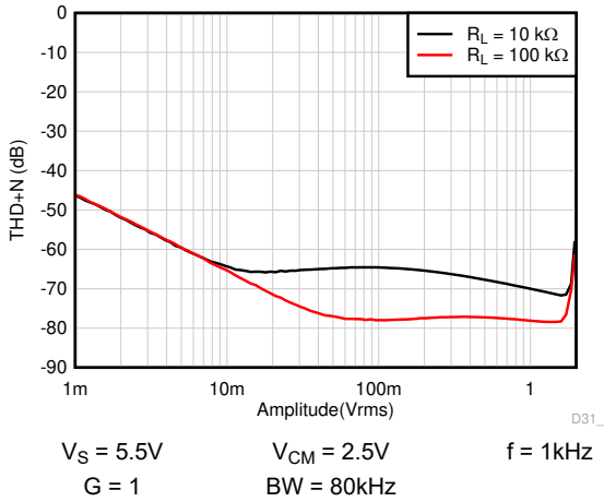
图 7-25. THD + N 与幅度间的关系
