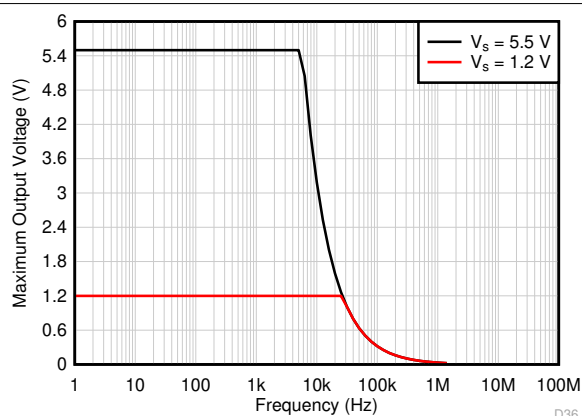
图 7-39. 最大输出电压与频率间的关系
