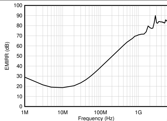
图 7-45. 以同相输入为基准的电磁干扰抑制比 (EMIRR+) 与频率间的关系
