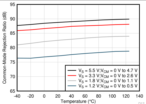
图 7-20. 直流 CMRR 与温度间的关系
