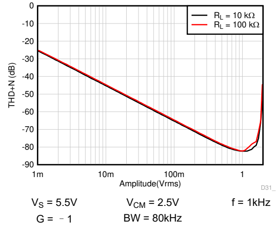
图 7-26. THD + N 与幅度间的关系
