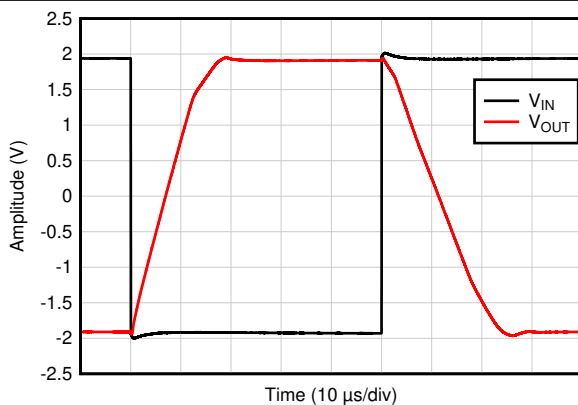
图 7-38. 大信号阶跃响应
