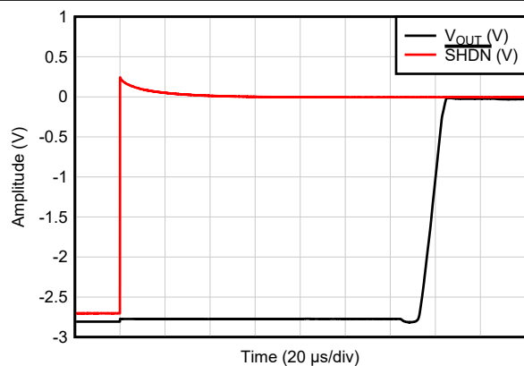
图 7-43. 放大器启用响应
