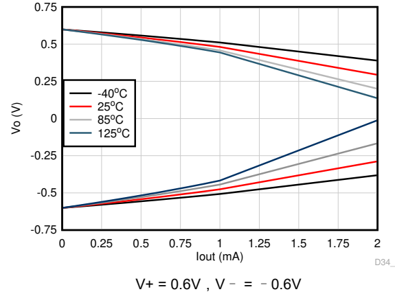
图 7-16. 输出电压与输出电流间的关系 ( 爪形 )
