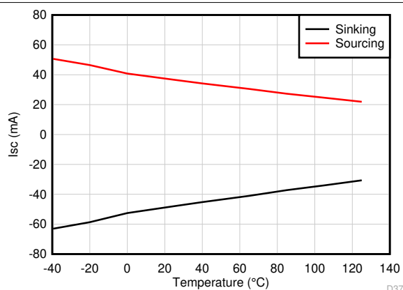
图 7-40. 短路电流与温度间的关系
