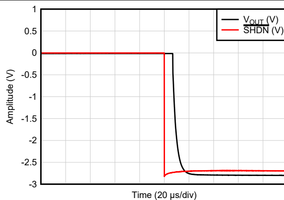
图 7-44. 放大器禁用响应
