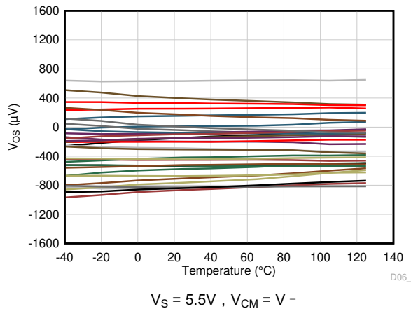
图 7-3. 输入失调电压与温度间的关系
