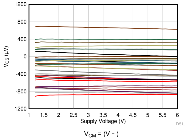
图 7-7. 偏移电压与电源电压间的关系
