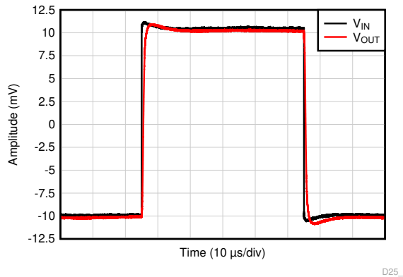
图 7-32. 无相位反转
