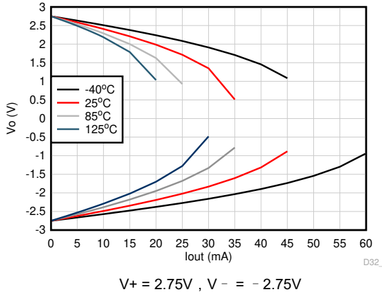
图 7-15. 输出电压与输出电流间的关系 ( 爪形 )
