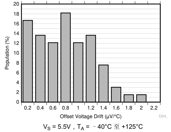
图 7-2. 失调电压漂移分布直方图
