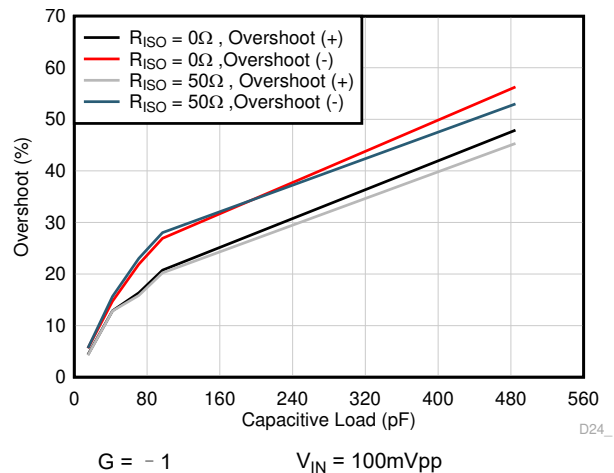
图 7-30. 小信号过冲与容性负载间的关系
