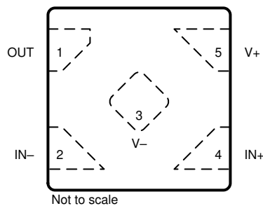
图 6-4. TLV9041 DPW 封装 5 引脚 X2SON 顶视图
