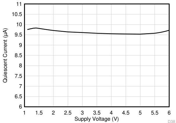
图 7-27. 静态电流与电源电压间的关系
