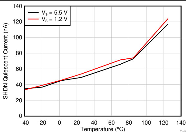
图 7-42. 关断模式静态电流与温度间的关系
