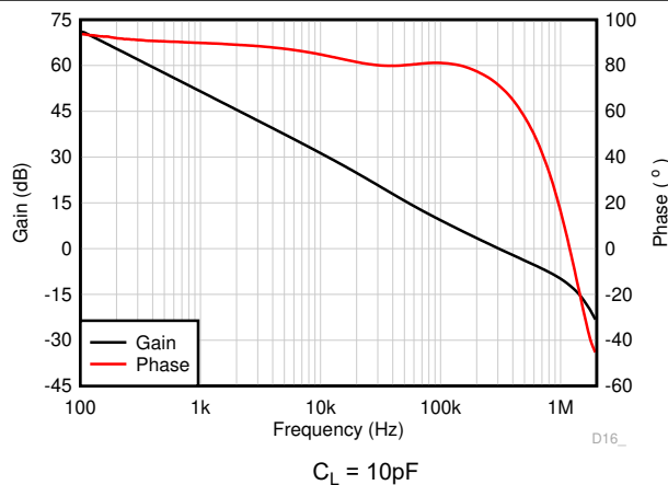
图 7-11. 开环增益和相位与频率间的关系
