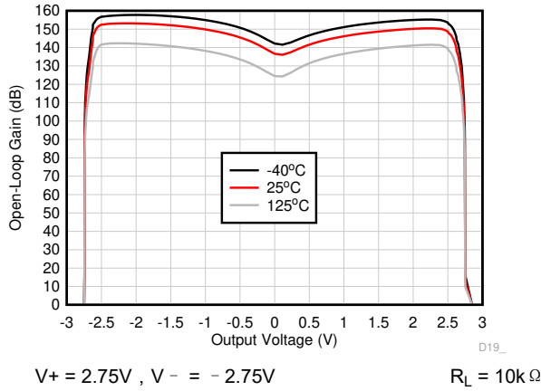
图 7-13. 开环增益与输出电压间的关系
