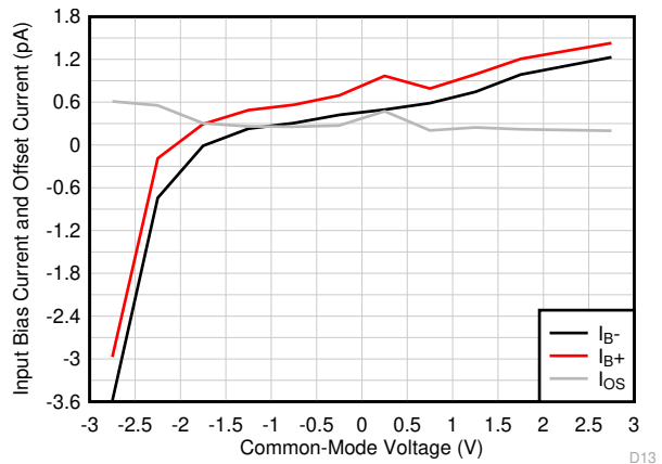
图 7-9. I_B 和 I_{OS} 与共模电压间的关系
