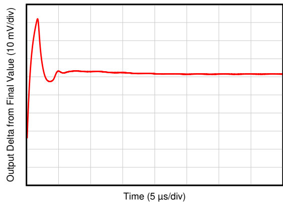
图 7-37. 大信号建立时间 ( 正 )
