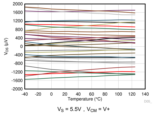
图 7-4. 输入失调电压与温度间的关系
