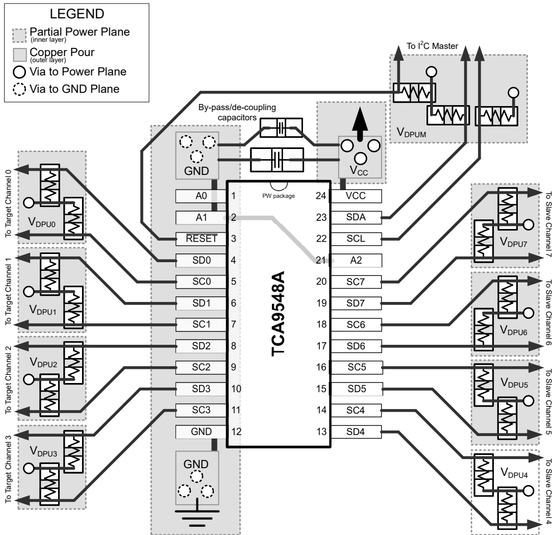
图 8-8. Layout Schematic
