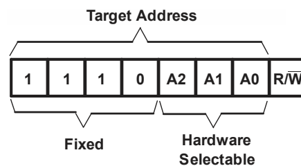
图 7-3. TCA9548A Address
