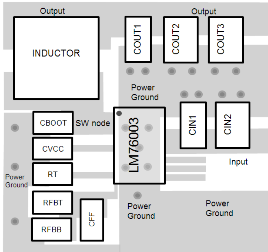
图 87. LM76002/LM76003 Layout
