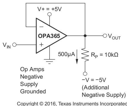
图 8-4. 摆动到接地
