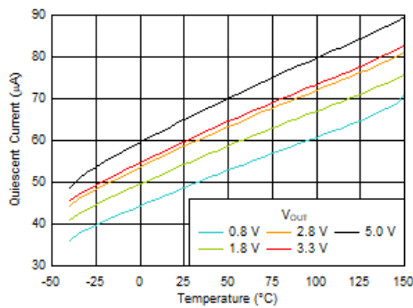
图 5-3. I_Q vs Temperature
