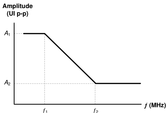
图 5-3. Input Jitter Tolerance Plot
