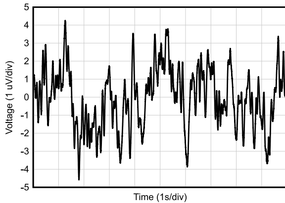
图 5-17. 0.1-Hz to 10-Hz Noise
