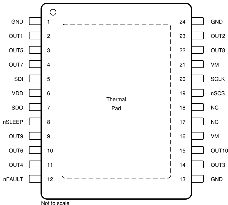
Pin Functions—DRV8910-Q1
