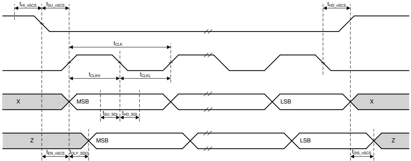
图 1. SPI Timing
