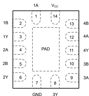
图 3-2. SN74LVC00A-Q1 BQA Package, 14-PIN WQFN (Top View)
