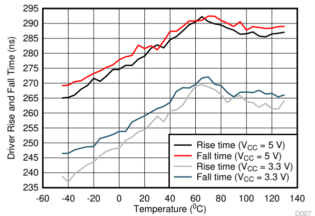
图 6-4. THVD2410 驱动器上升时间或下降时间与温度之间的关系
