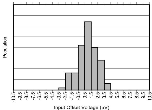
图 6-2. INA241A2-Q1 输入失调电压产生分布图
