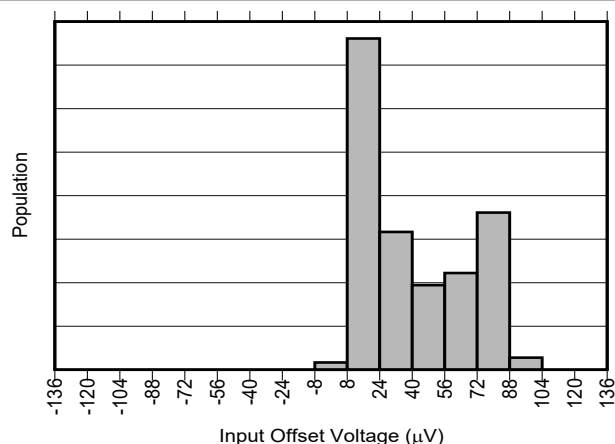
图 6-3. INA241A3-Q1 和 INA241A4-Q1 输入失调电压产生分布图
