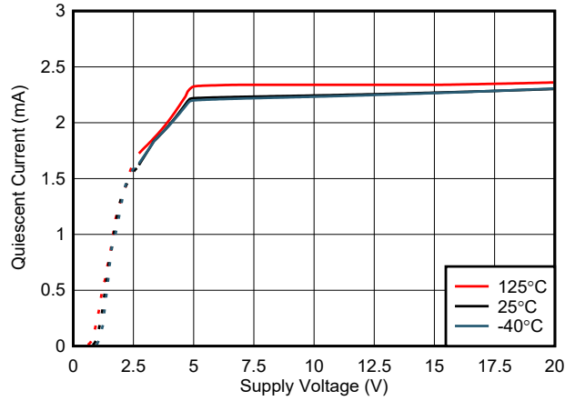
图 6-31. 静态电流与电源电压间的关系
