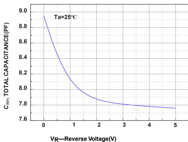
Fig 3. C_{TOT}-V_R
