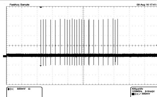
图 7-19. 10BASE-T Link Pulse Waveform
