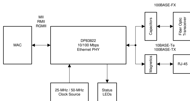
简化原理图
