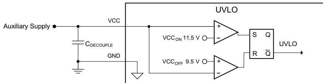
图 24. UVLO
