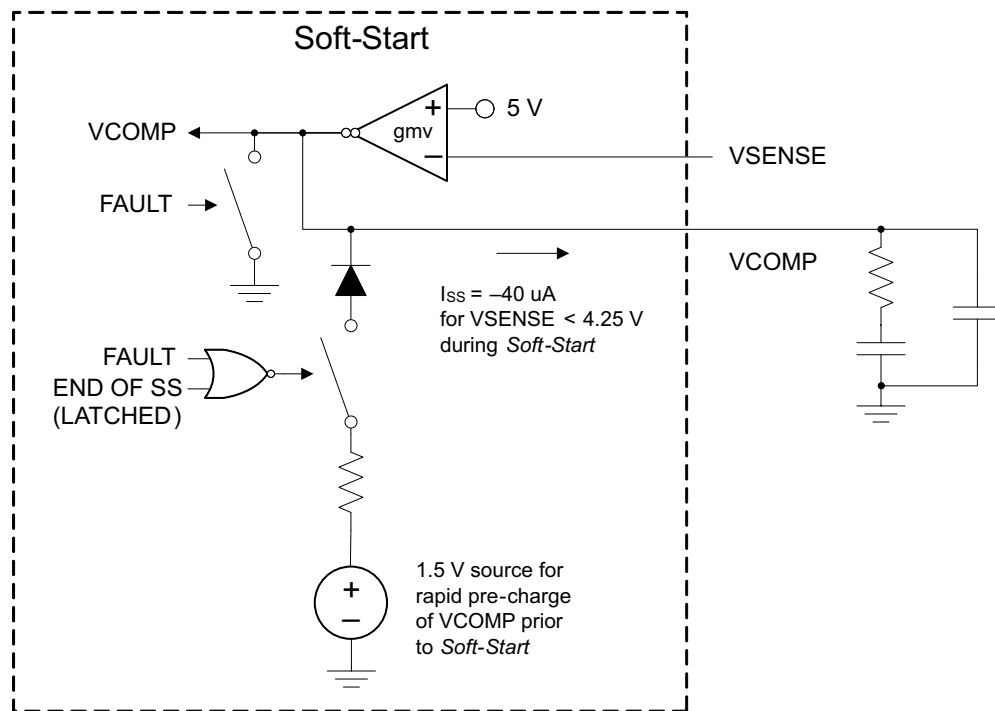
图 23. Soft Start
