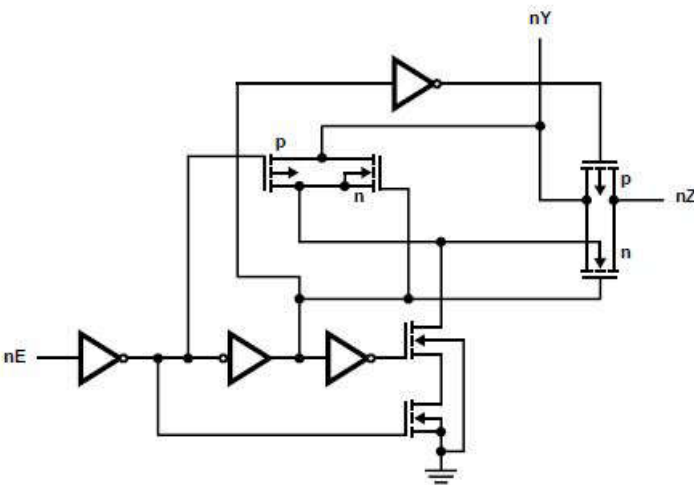
图 16-2. Logic Diagram
