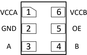
图 4-1. DRY 封装
