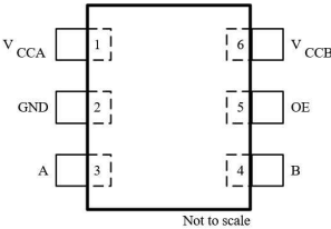
图 4-2. DBV、DCK 和 DRL 封装
