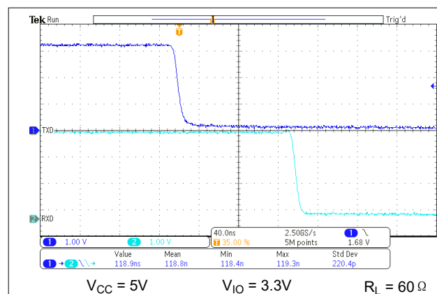
图 8-4. t_{PROP(LOOP1)}
