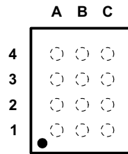
图 4-1. GXU 和 ZXU 封装，12 引脚 BGA Microstar Junior (顶视图)
