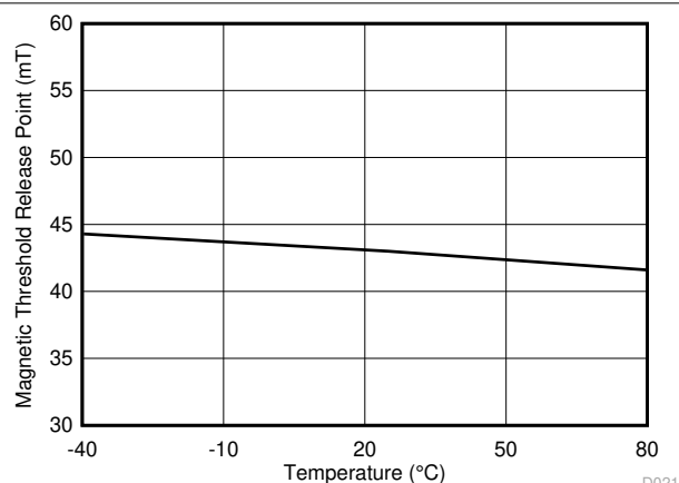
图 6-9. ZE 版本 |B_{RP}| 与温度间的关系
