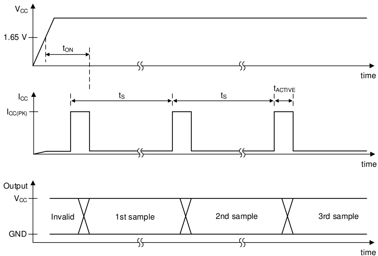
图 7-7. 时序图
