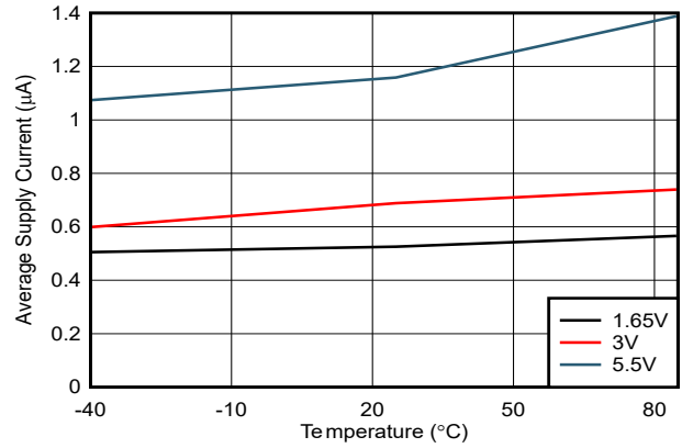
图 6-2. I_{CC(AVG)} 与温度间的关系 (5Hz 版本)
