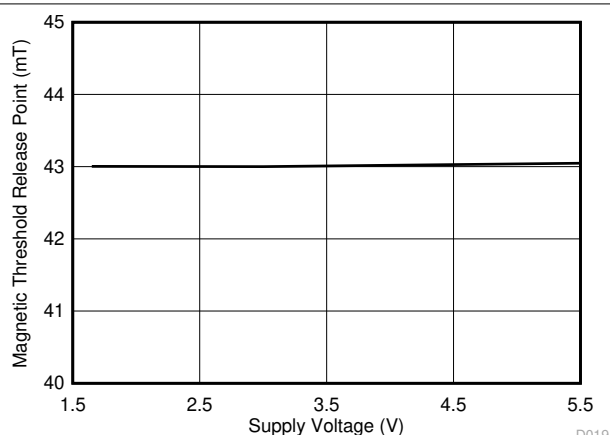
图 6-11. ZE 版本 |B_{RP}| 与 V_{CC} 间的关系
