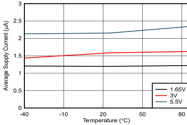
图 6-1. I_{CC(AVG)} 与温度间的关系 (20Hz 版本)
