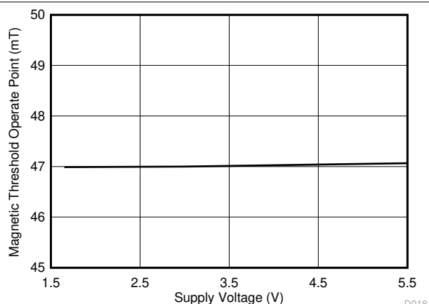
图 6-10. ZE 版本 |B_{OP}| 与 V_{CC} 间的关系
