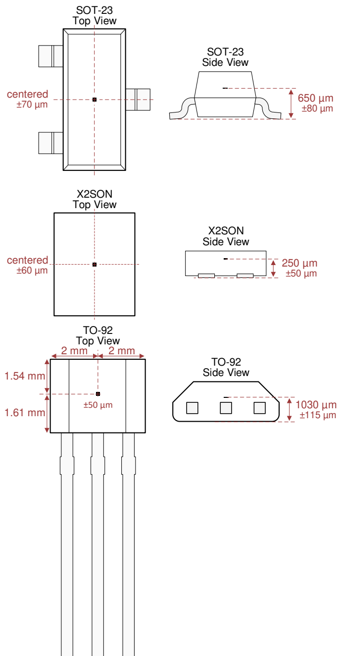
图 7-8. 霍尔元件位置
