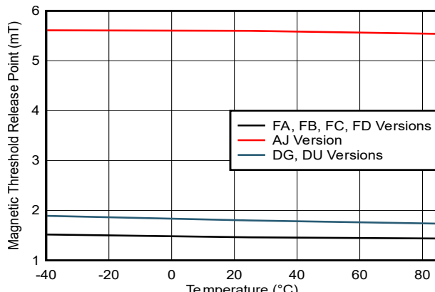
图 6-5. |B_{RP}| 与温度间的关系
