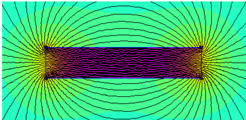
图 8-5. 典型磁通线
