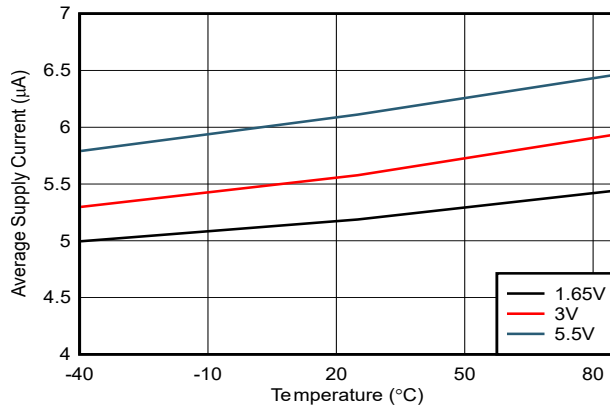
图 6-3. I_{CC(AVG)} 与温度间的关系 (40Hz 版本)
