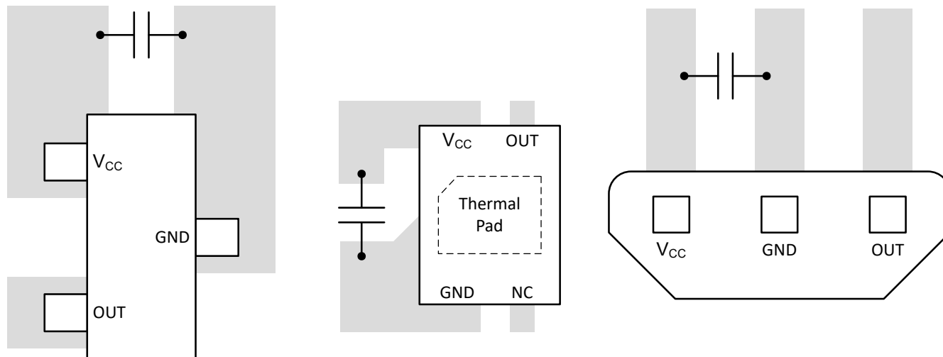
图 8-7. 布局示例
