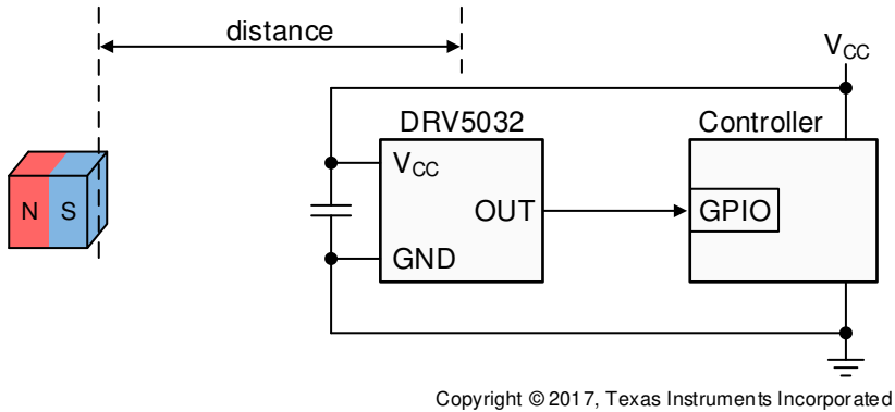
图 8-1. 典型应用图
