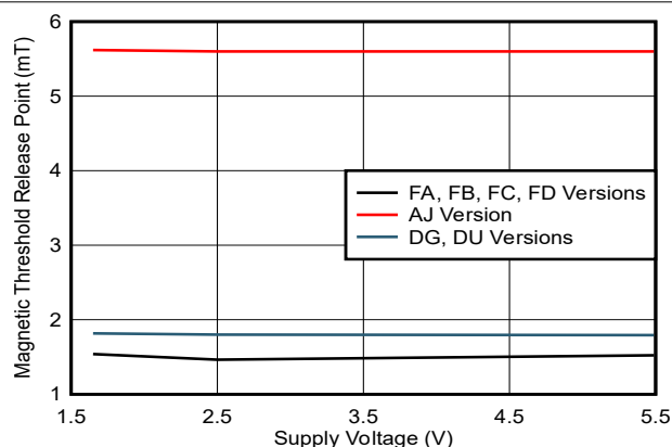
图 6-7. |B_{RP}| 与 V_{CC} 间的关系
