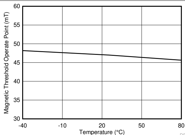
图 6-8. ZE 版本 |B_{OP}| 与温度间的关系
