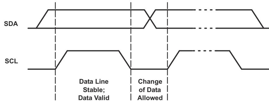
图 8-2. Bit Transfer
