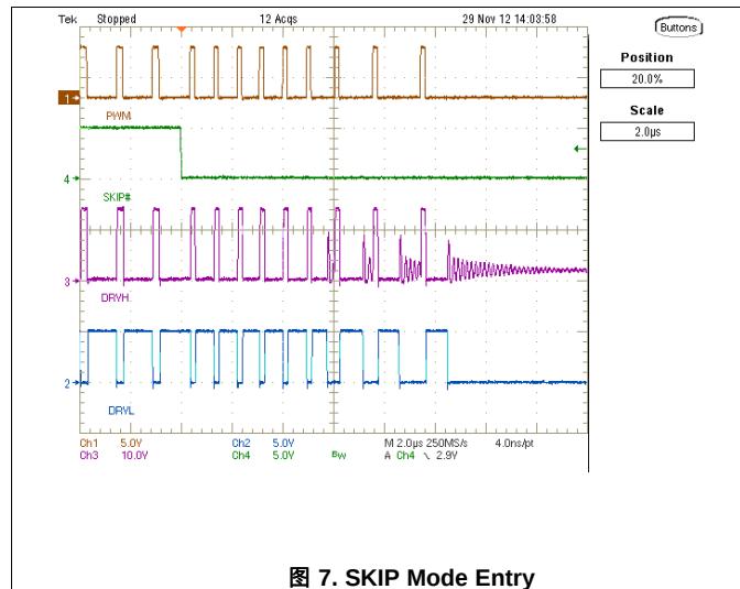
图 7. SKIP Mode Entry
