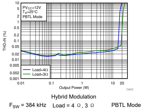
图 7-29. THD+N vs Output Power-PBTL
