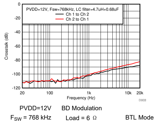
图 7-59. Crosstalk
