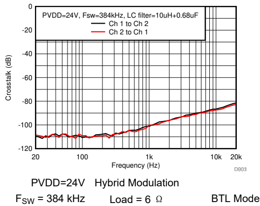
图 7-19. Crosstalk
