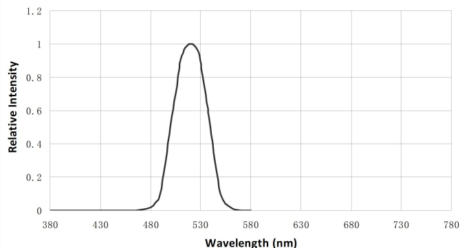
光谱分布特性曲线 Spectrum Distribution ( T_a=25^\circ\text{C} )
