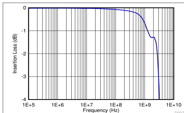
图 5-7. Insertion Loss
