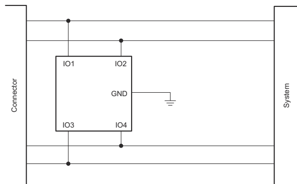
简化原理图
