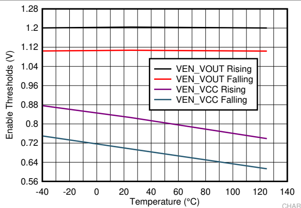
图 7-8. Enable Thresholds
