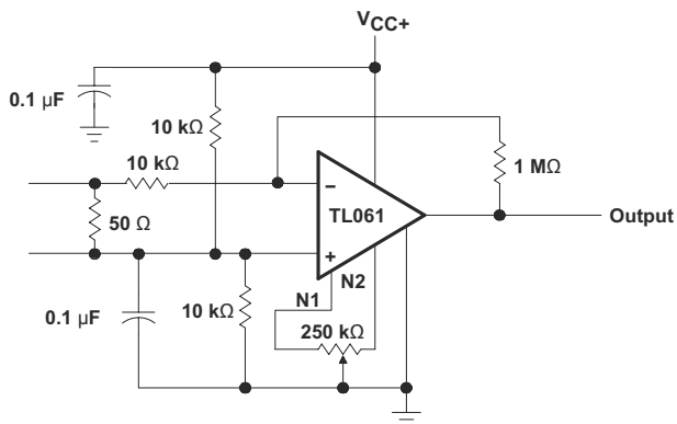
图 9-8. AC Amplifier
