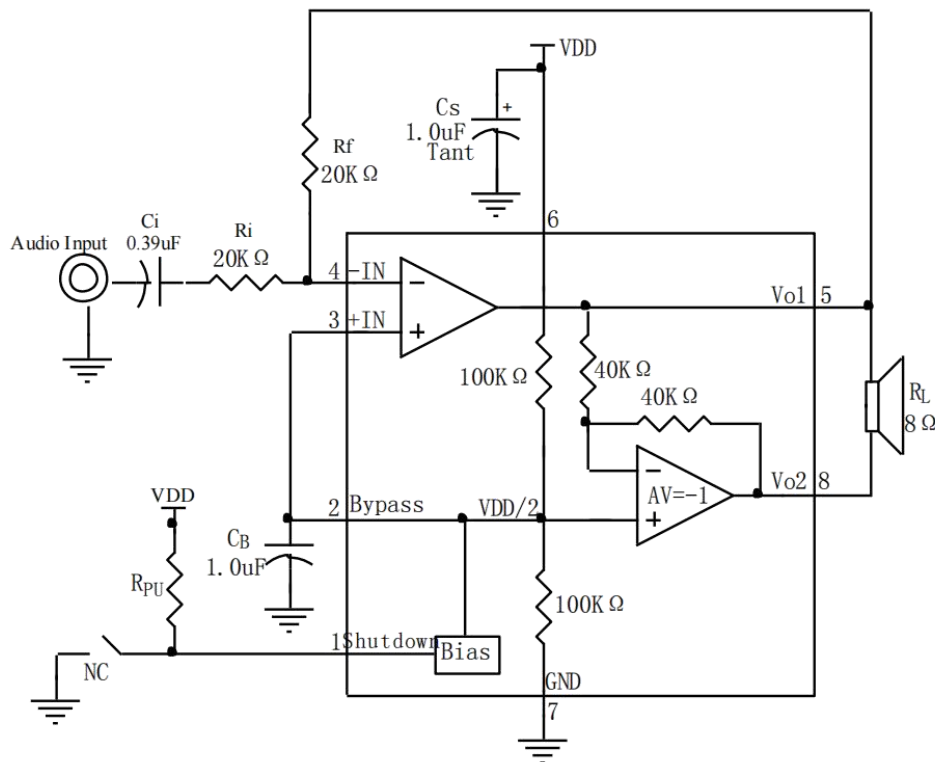
图 1、LM4871B 典型应用图
