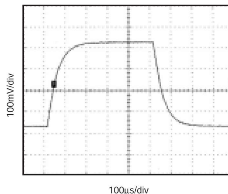
图 5-12. 小信号阶跃响应 - G = 100
