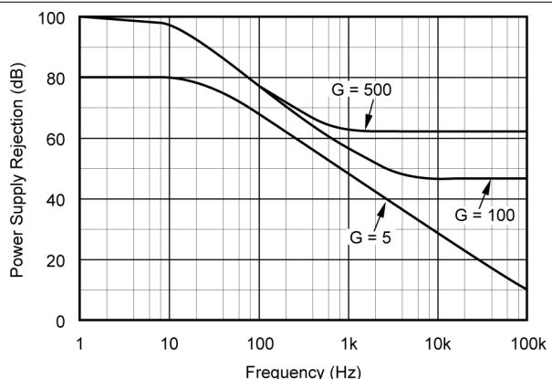
图 5-4. 负电源抑制与频率间的关系
