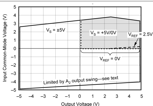
图 6-4. 输入共模范围与输出电压间的关系， V_S = \pm 5 ， G = 5
