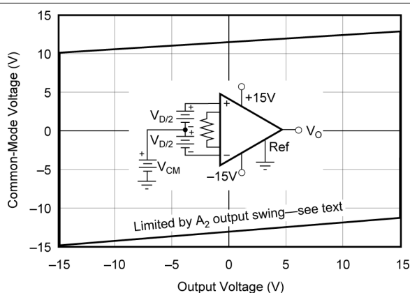
图 6-3. 输入共模范围与输出电压间的关系， V_S = \pm 15V ， G = 5
