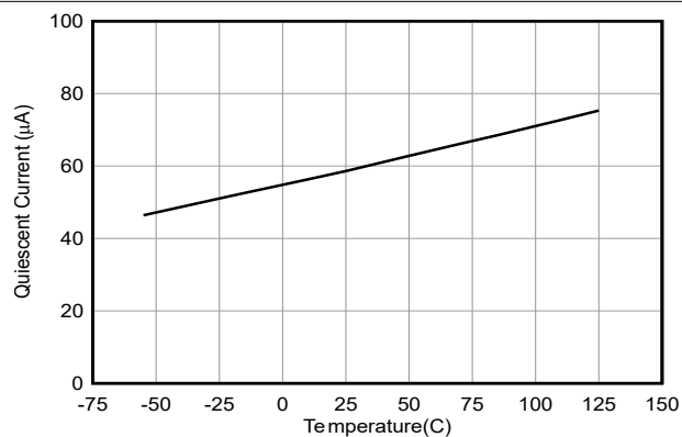
图 5-8. 静态电流与温度间的关系
