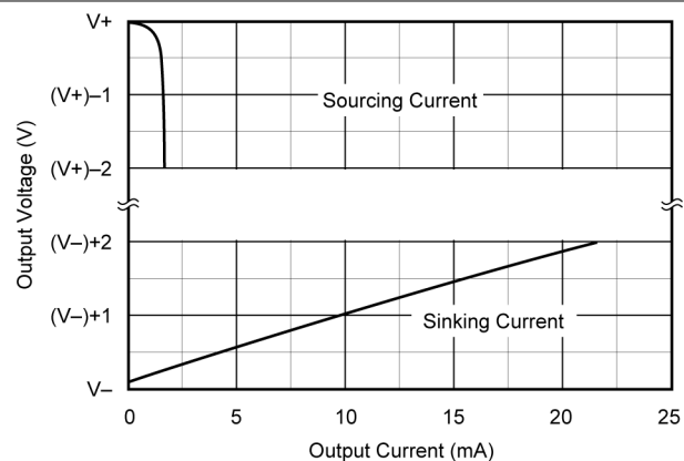
图 5-10. 输出电压摆幅与输出电流间的关系
