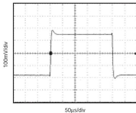
图 5-11. 小信号阶跃响应 - G = 5
