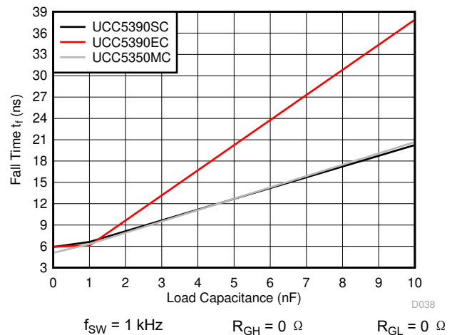
图 6-40. Fall Time vs Load Capacitance
