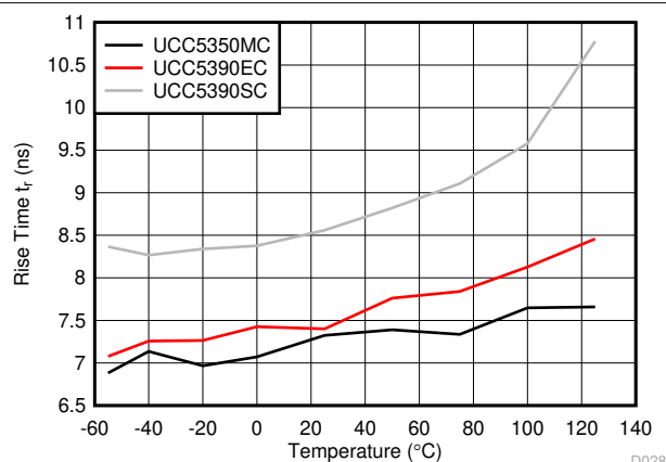
图 6-28. Rise Time vs Temperature
