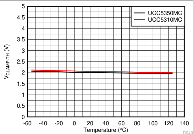
图 6-26. V_{Clamp-TH} vs Temperature
