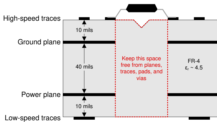
图 11-5. Recommended Layer Stack
