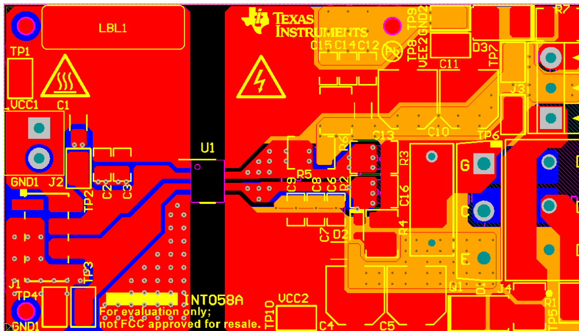
图 11-1. Layout Example
