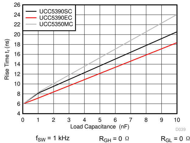
图 6-37. Rise Time vs Load Capacitance
