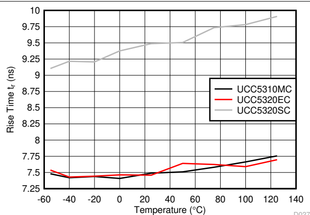
图 6-27. Rise Time vs Temperature
