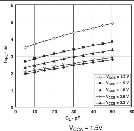
图 6-4. 典型传播延迟 (A 至 B) 与负载电容间的关系
