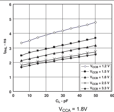
图 6-6. 典型传播延迟 (A 至 B) 与负载电容间的关系
