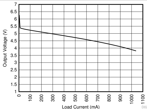
图 6-23. Output Voltage vs Load Current
