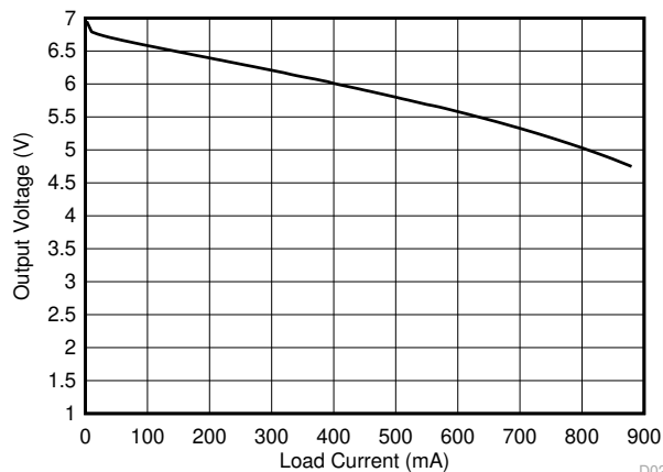
图 6-25. Output Voltage vs Load Current
