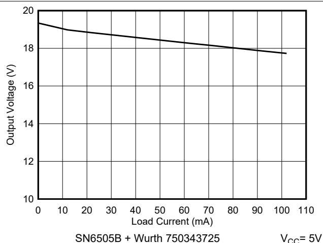
图 6-37. Output Voltage vs Load Current
