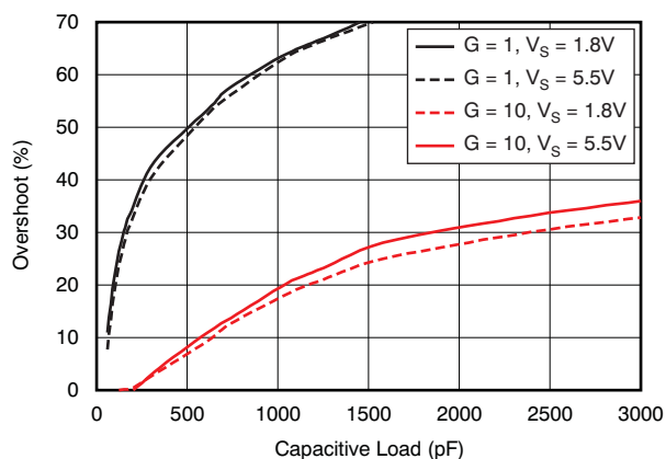
图 37. 小信号过冲与容性负载间的关系 (100mV pp 输出阶跃)
