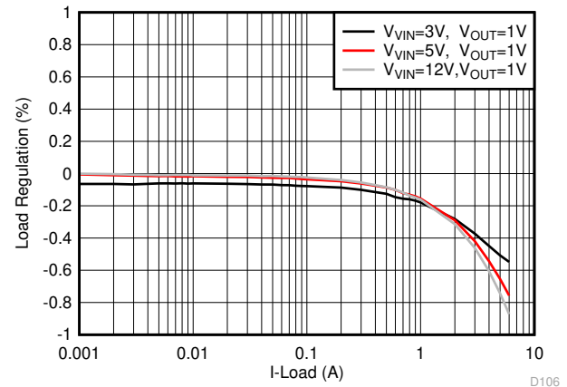
图 7-5. TPS566238 Load Regulation
