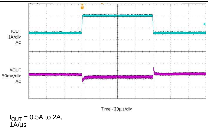
图 27. Load Transient
