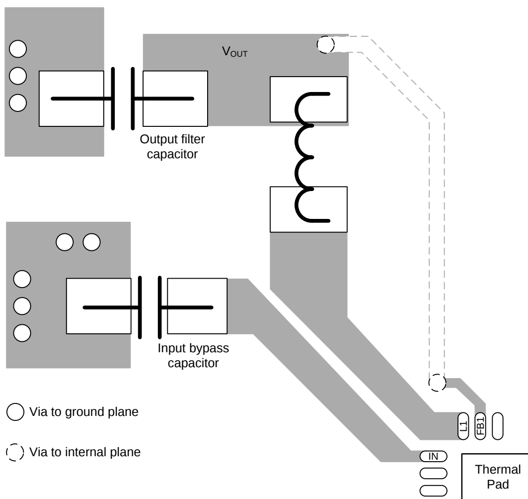
图 78. Layout Example Schematic
