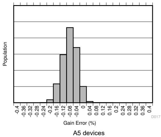
图 6-7. Gain Error Production Distribution
