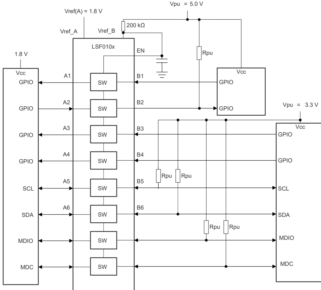
图 9-4. 使用 LSF010x-Q1 进行多电压转换
